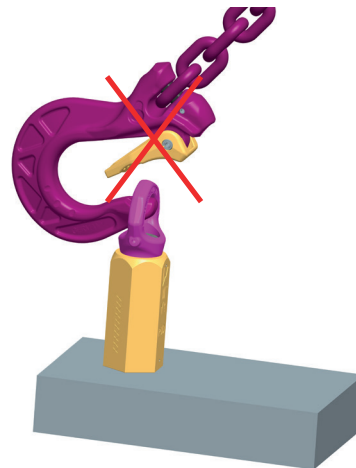
Abb. 2: Verwenden Sie nur passende Anschlagmittel zum Einhängen in die VRS mit Sechskant-Verlängerungsadapter
