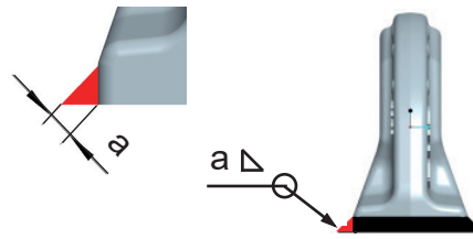
Abb. 4: Schweißnahtanordnung
