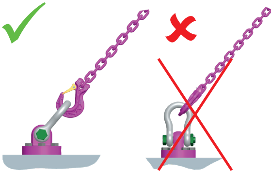
Abb. 1: Richtig! In Krafrichtung ausgerichtet
