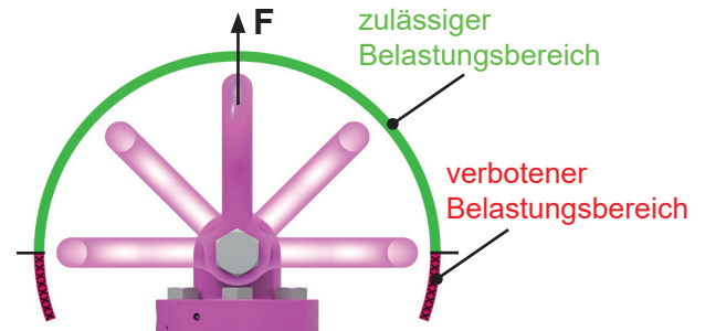
Abb. 5: Schwenken in Klapprichtung (grün = zulässiger Belastungsbereich)
